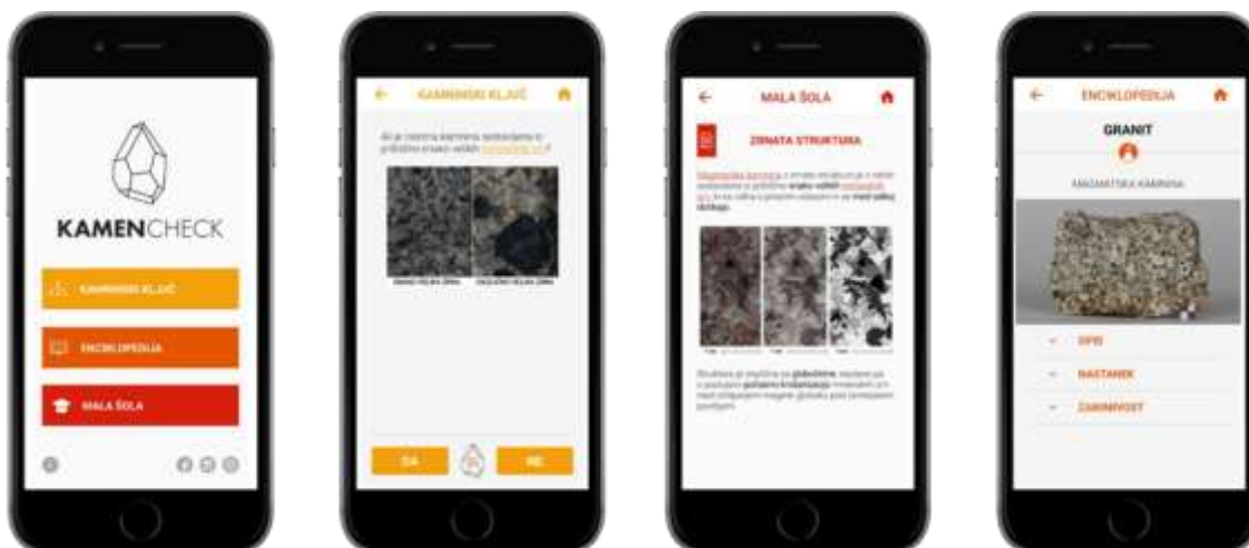
Slika 8: Aplikacija KamenCheck.
