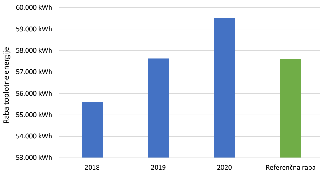
Graf 2.2: Dejanska in referenčna raba toplotne energije
