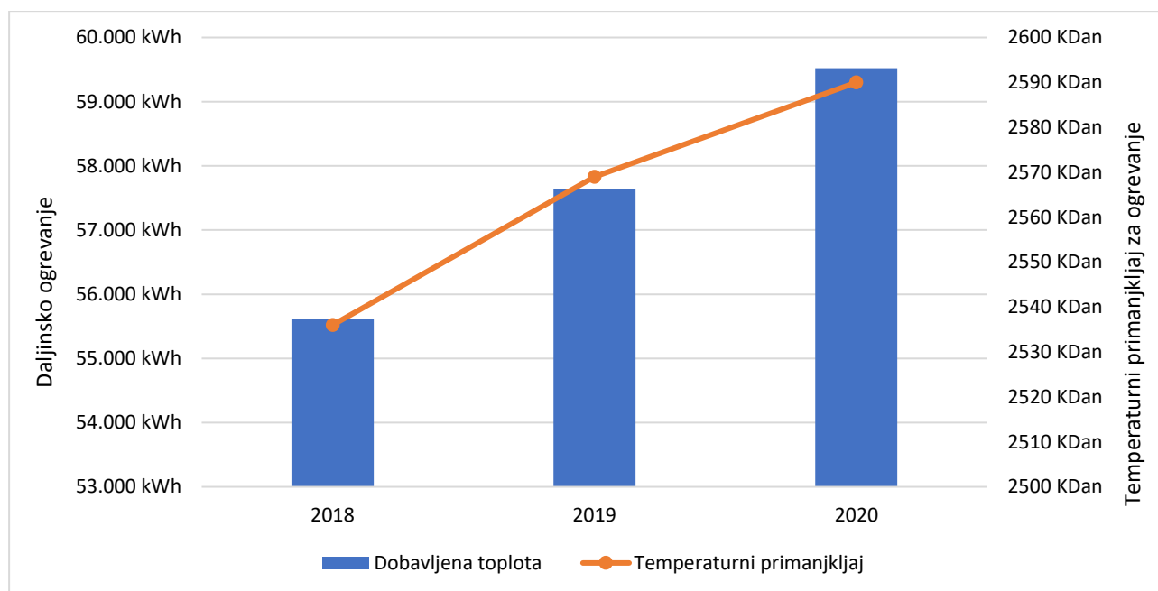
Graf 4.11: Letna raba toplotne energije in temperaturni primanjkljaj
