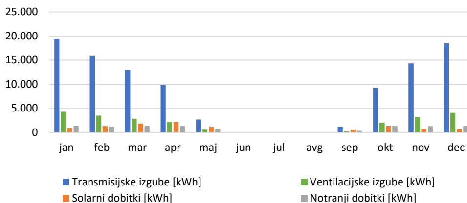
Graf 8.1: Prikaz izračunanih mesečnih toplotnih izgub in dobitkov – (hipotetično) obstoječe stanje
