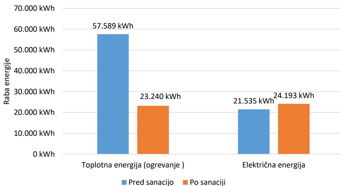
Slika 0.1: Primerjava (hipotetične) rabe energije pred in po izvedeni celoviti prenovi
